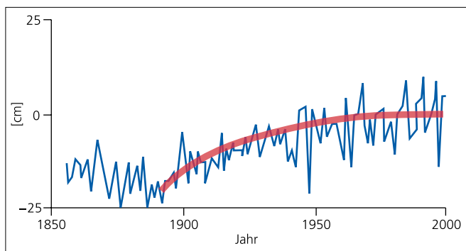
Abb. 4. Pegelstandsmessungen in Cuxhaven von 1850 bis 2000.
